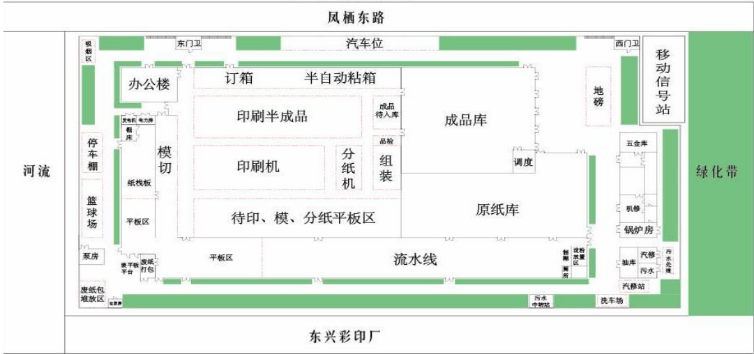
浙江济丰包装纸业有限公司 厂区平面图
